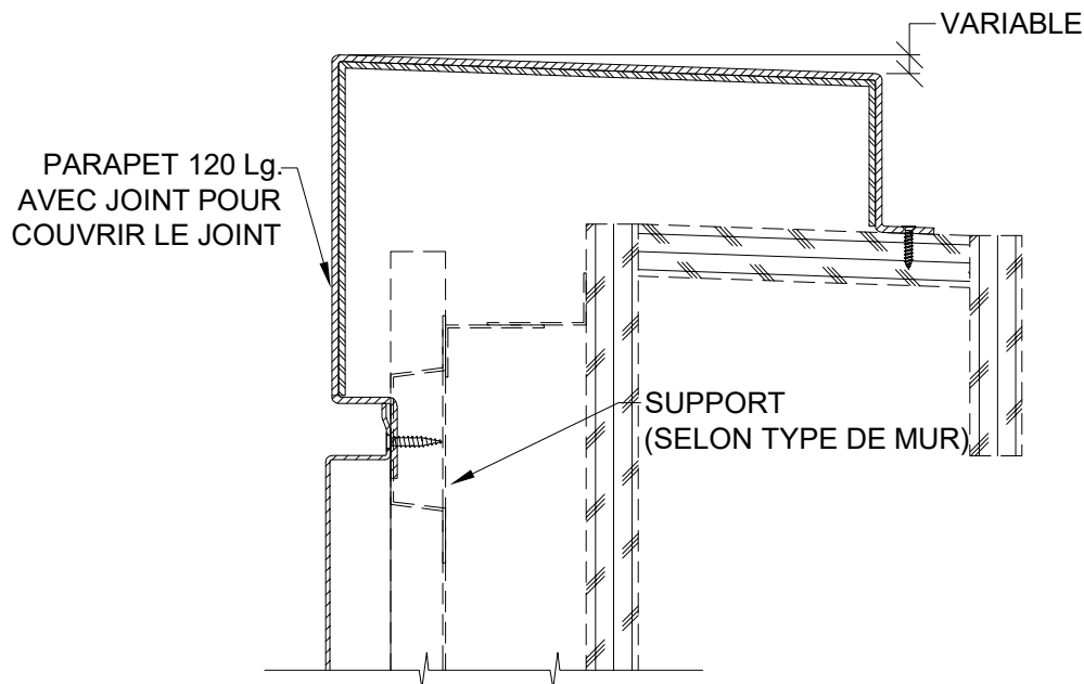
DÉTAIL PARAPET (VUE EN ÉLÉVATION)
