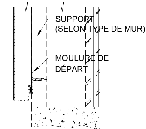
DÉTAIL PANNEAU DE DÉPART (VUE EN ÉLÉVATION)
